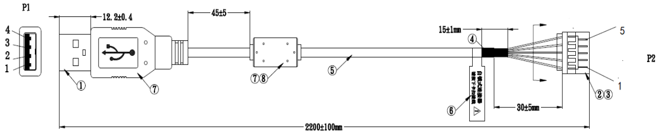
接点图
